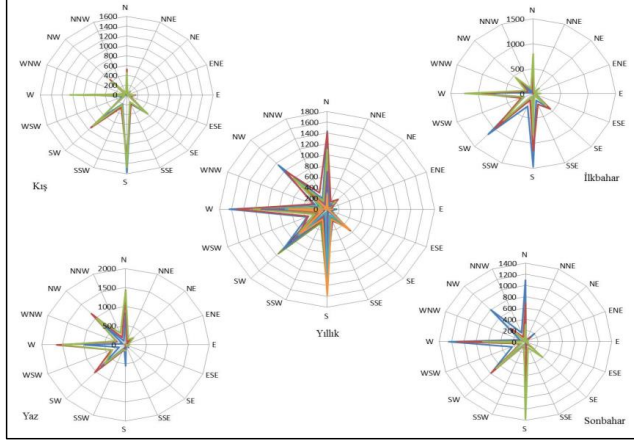
Şekil 3: Mesudiye Hakim Rüzgar Yönü ve Rüzgar Gülleri.
