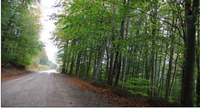
Foto 23: Kozören Çevresinde Dağılış Gösteren Saf Kayın ( fagus orientalis ) Ormanları.
