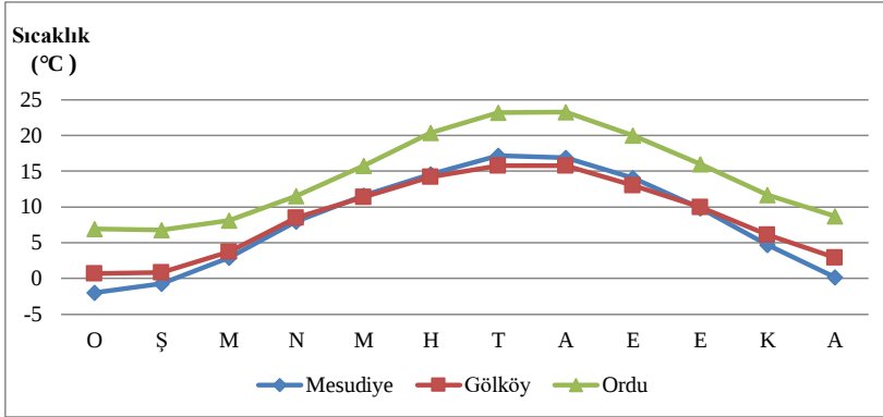
Grafik 2: Ordu-Mesudiye ve Gökçöy İstasyonlarına Ait Termik Rejim Diyagramı (MGM).
