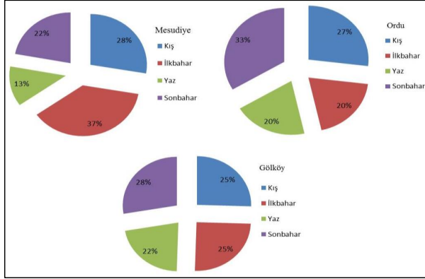
Grafik 7: Ordu, Mesudiye ve Gökçöy’de Yağışın Mevsimlere Göre Dağılışı.
