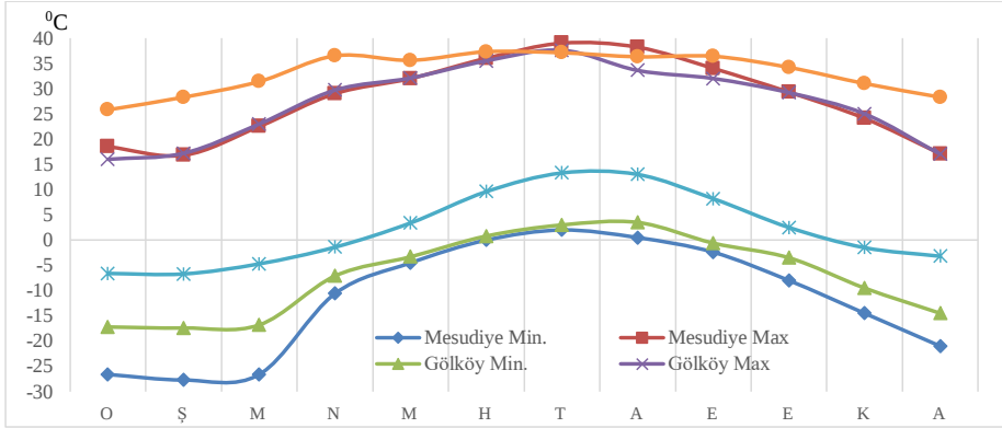
Grafik 3: Ordu, Gölköy ve Mesudiye İstasyonlarının Mutlak Maksimum ve Mutlak Minimum Sıcaklık Karşılaştırması.
