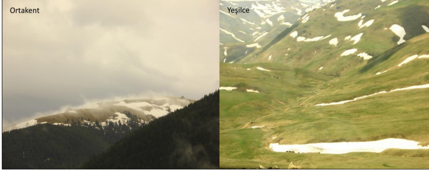
Foto 28: Ortakent ve Yeşilce Çevresinde Geniş Sahalara Yayılan Alpin Çayırları.
