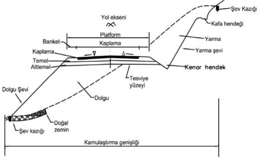
Şekil 3. 1. Bölünmemiş (tek platformlu) bir yola ait enkesit.
