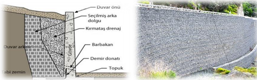
Şekil 3. 4. Betonarme istinat duvarı modellemesi ve istinat duvarı inşası.
