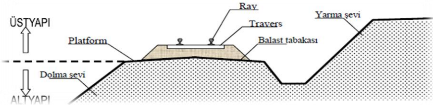
Şekil 3. 9. Demiryolunun bölümleri.
