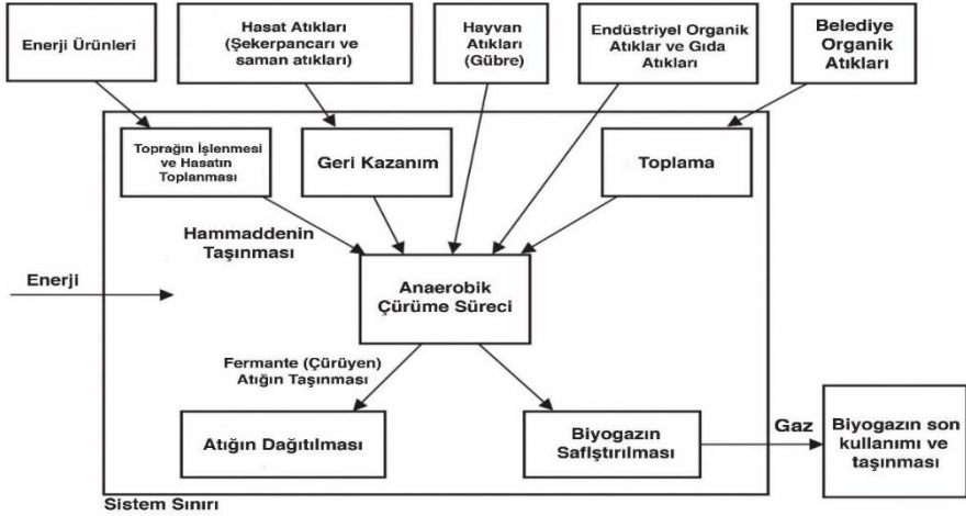
Şekil 1: Biyogaz Üretim Sisteminde Hammadde ve Enerji Akışları Diyagramı 3 .
