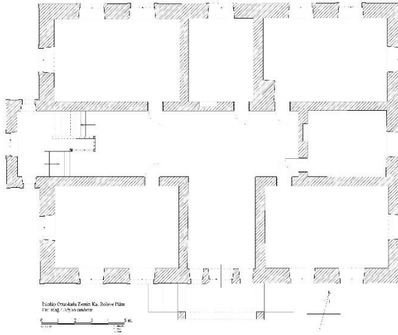
Plan 3: Emirdağ Merkez İnkılâp Ortaokulu Zemin Kat Röleve Planı
