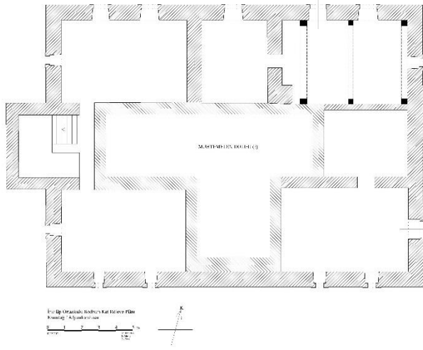
Plan 2: Emirdağ Merkez İnkılâp Ortaokulu Bodrum Kat Röleve Planı
