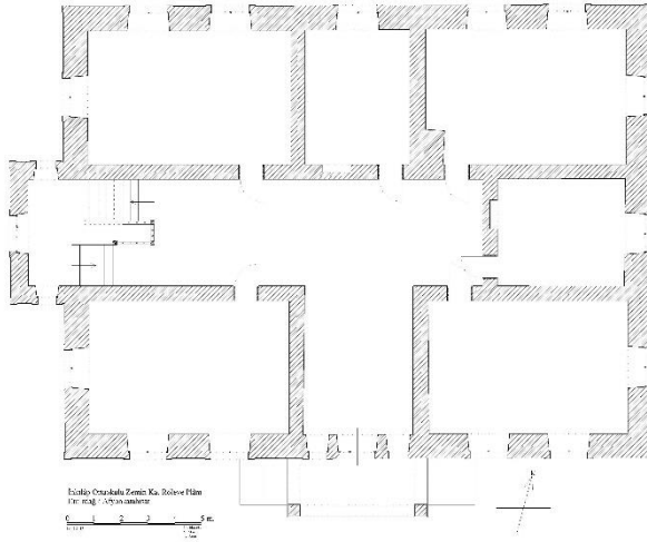
Plan 3: Emirdağ Merkez İnkılâp Ortaokulu Zemin Kat Röleve Planı
