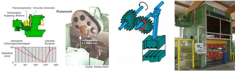
Şekil 17. Dairesel olmayan dişlilerin pres makinelerinde kullanımı
