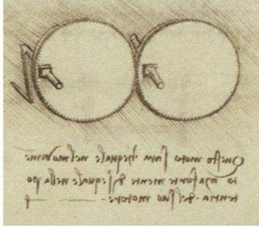
Şekil 4. Dairesel olmayan bir dişli çifti tarafından sürekli bir dönme hareketinin aktarılmasının ilk gerçek örneği
