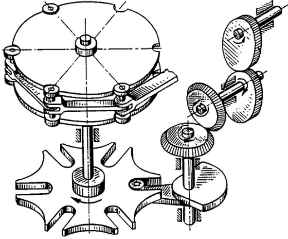
Şekil 9. Genova Mekanizması
