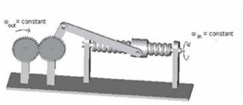
Şekil 16. Krank biyel mekanizması
