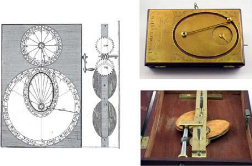
Şekil 5. Desagulier'in kuyruklu yıldızı iki eliptik makara
