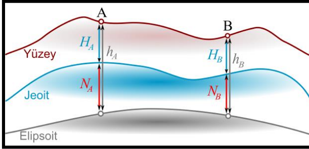
Şekil-5 Fiziksel yeryüzü, jeoit ve elipsoit arasındaki ilişki (Türen, 2010).
