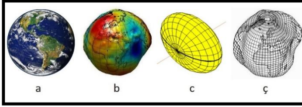
Şekil-4 Küresel konumlama sistemlerinden elde edilen yatay ve düşey koordinat bileşenlerinin elde edilmesinde kullanılan yeryuvarına ait yüzeyler;
