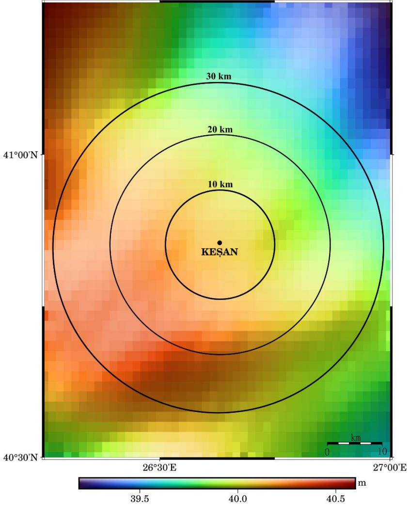
Şekil-7 Uygulamaya yönelik çalışma sahasının jeoit ondülasyonu görünümü.
