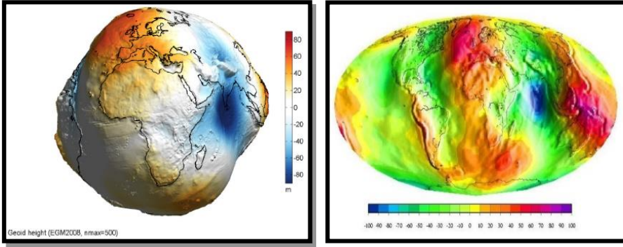
Şekil-3 Yerçekimi alanı modeli EGM2008'den hesaplanan jeoit yüksekliklerin farklı renk skalasında üç boyutlu ve iki boyutlu görünümü (Pavlis, vd., 2012).
