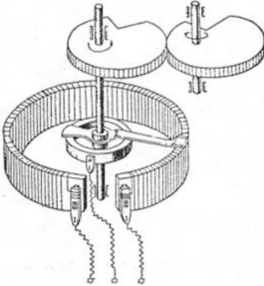
Şekil 8. Potansiyometre
