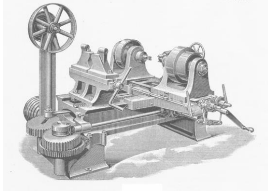
Şekil 13. Kanal açma makinesi
