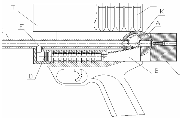
Şekil 12. Şarjör mekanizmasında dairesel olmayan dişli kullanımı
