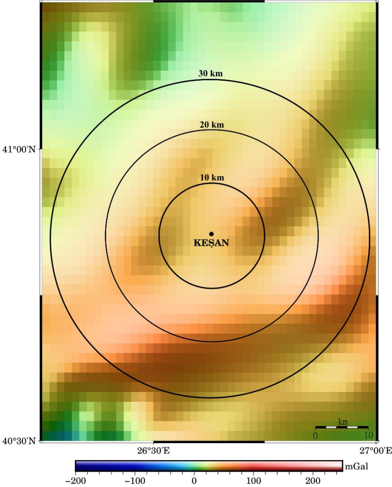
Şekil-8 Uygulamaya yönelik çalışma sahasının serbest gravite anomalisi görünümü.
