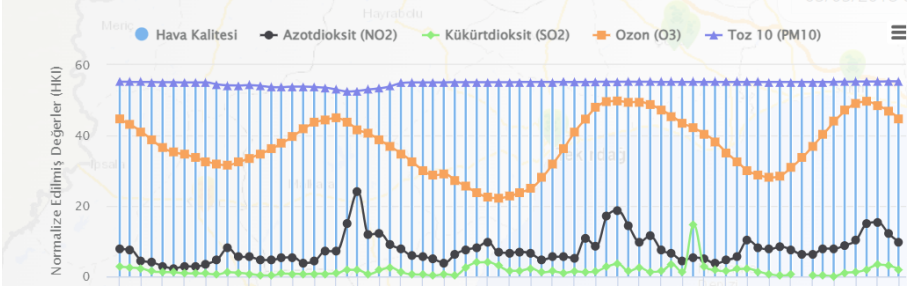
Şekil 3.1: 2018 Mayıs ayı Keşan ilçesi Hava Kirliliği Özeti [14]
