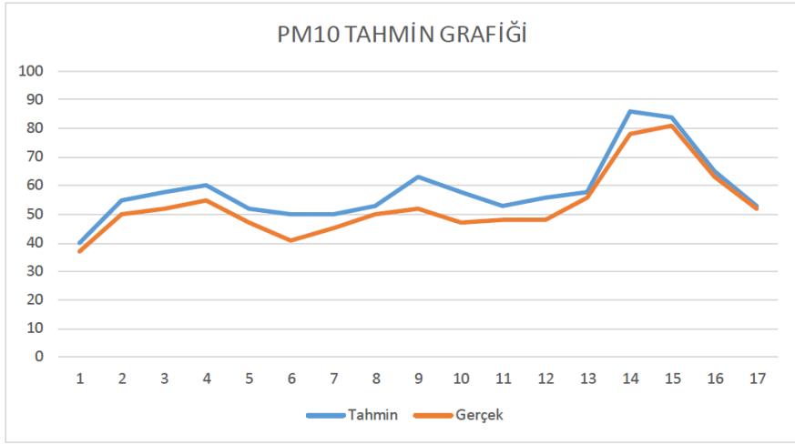
Şekil 2.7: 2018 yılı PM10 Tahmin Grafiği
